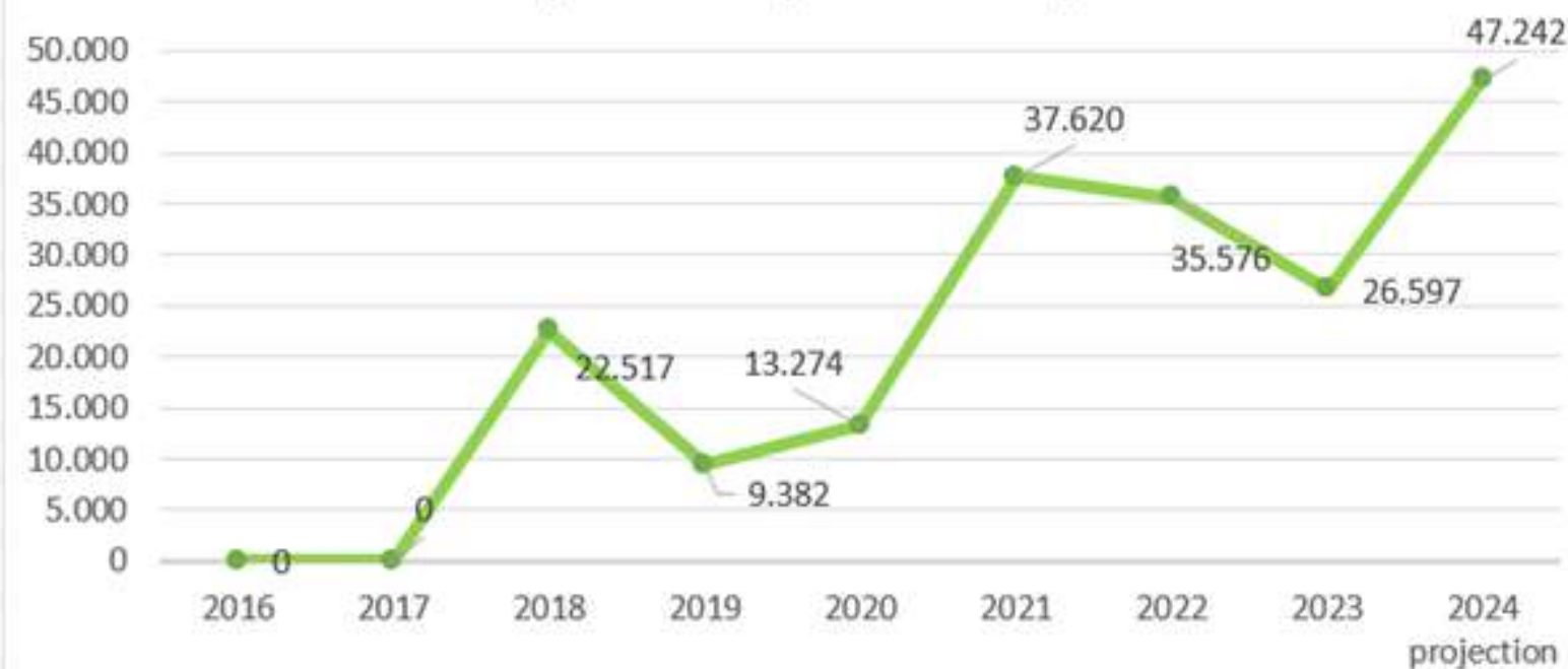
Graphe 5 : Economie d'énergie (en KWh) - Installation des panneaux photovoltaïques
